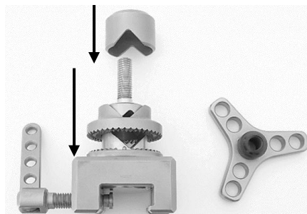
Fig. 2: Morsetto di fissaggio per tavolo operatorio EEJ-1 (a titolo esemplificativo)
