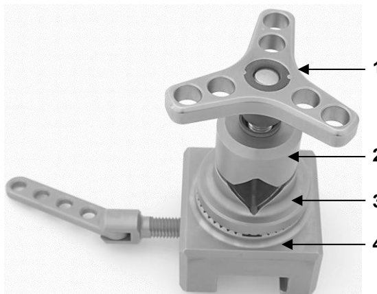
Fig. 2: Morsetto di fissaggio per tavolo operatorio EEJ-1 (a titolo esemplificativo)
