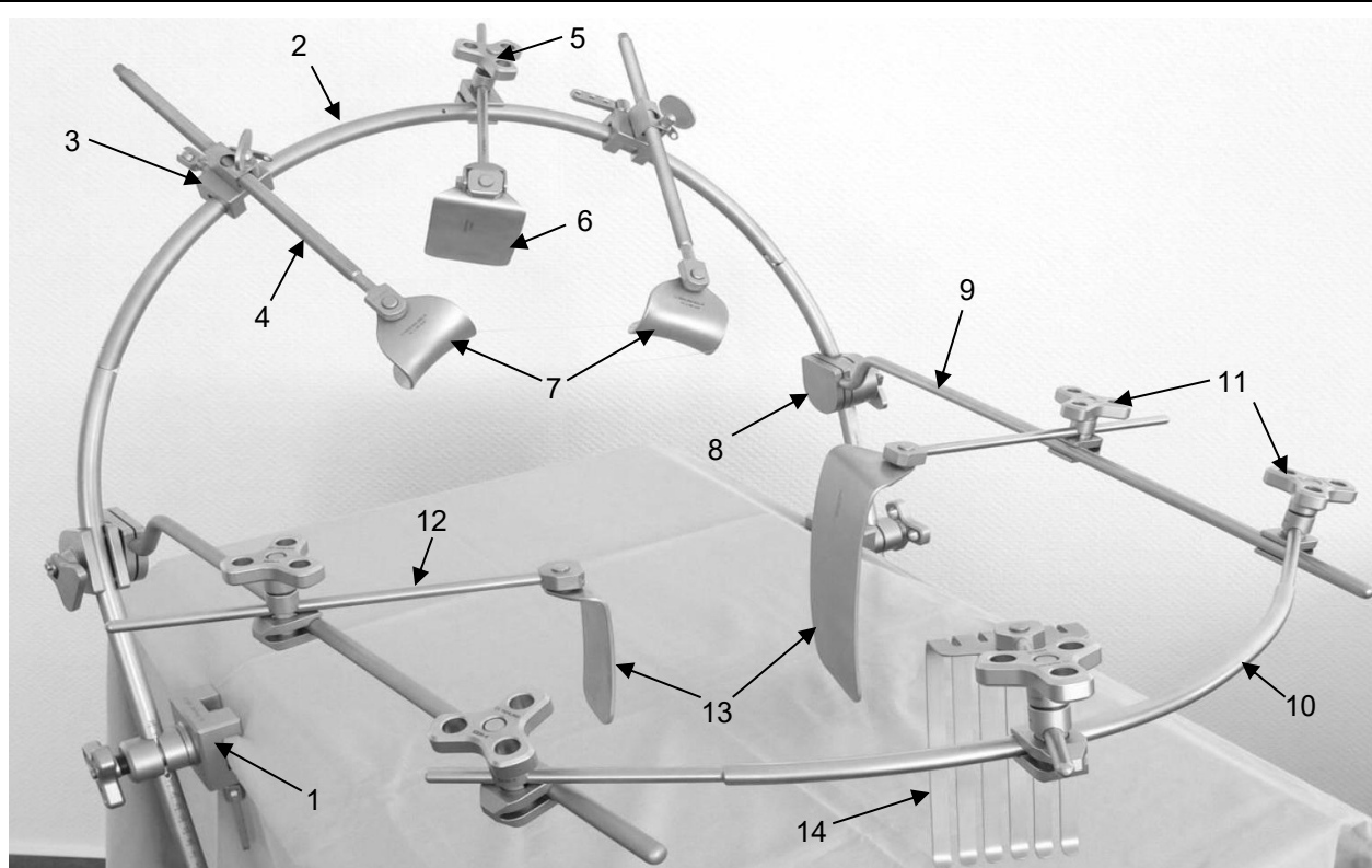
Fig. 1: Esempio di configurazione del sistema di retrazione VENTREXPO
