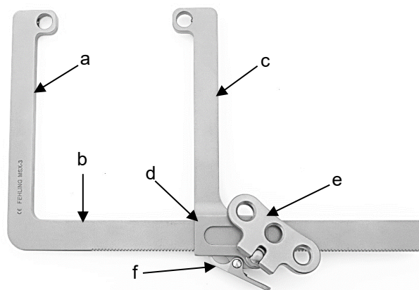
Afb. 3: Voorbeeld van een U-vormige balkspreider met tandwiel/vergrendeling
