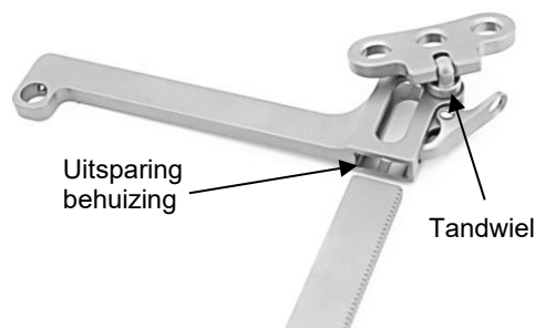
Afb. 3: Voorbeeld van een U-vormige balkspreider met tandwiel/vergrendeling
