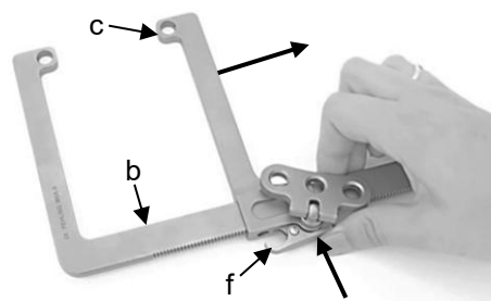
Afb. 11: Voorbeeld van een U-vormige balkspreider met tandwiel/vergrendeling
